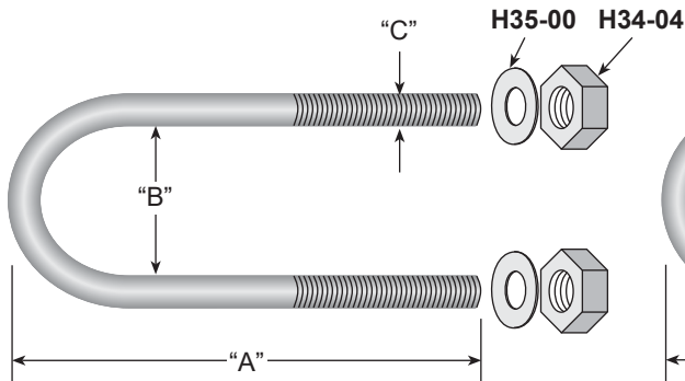
U-BOLT "KIT"
