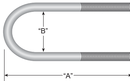
U-BOLT
