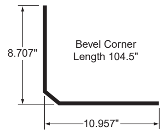
CORNER LINER, FRUEHAUF, GALV
