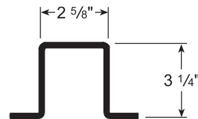
OFFSET BOTTOM
